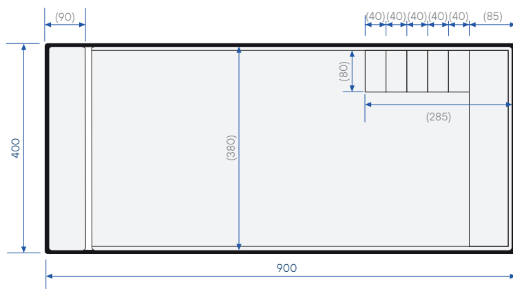
Sicht von oben
