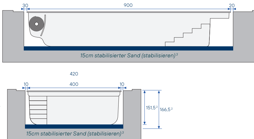
Sicht von der Innenseite des Pools
