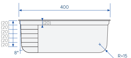
Sicht von der Innenseite des Pools
